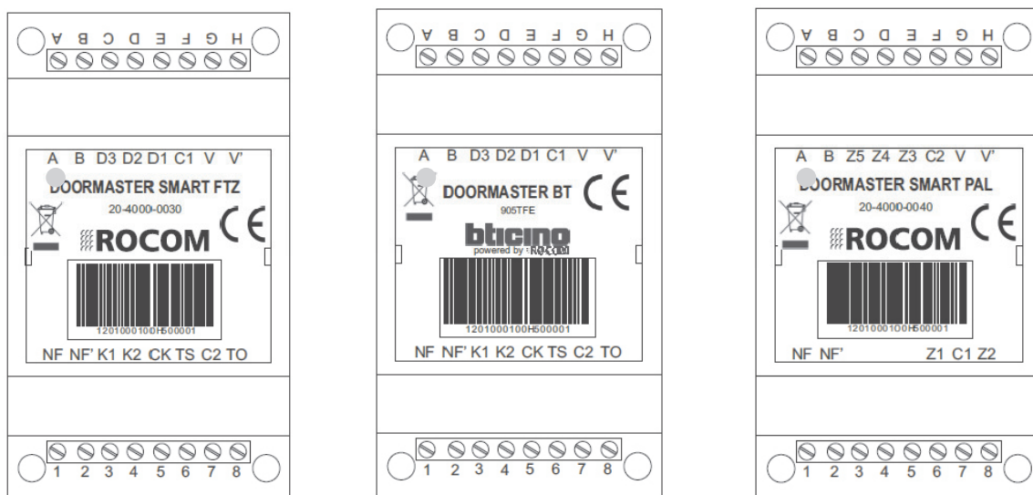
Anschlussklemmen Doortello Smart FTZ, BT und PAL
