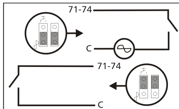
Brückensteckereinstellung für potentialfreie Klingeltasten
