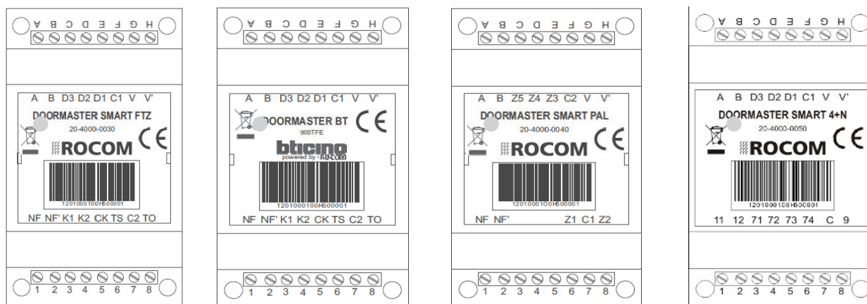
Anschlussklemmen Doortello Smart FTZ, BT, PAL und 4+N
